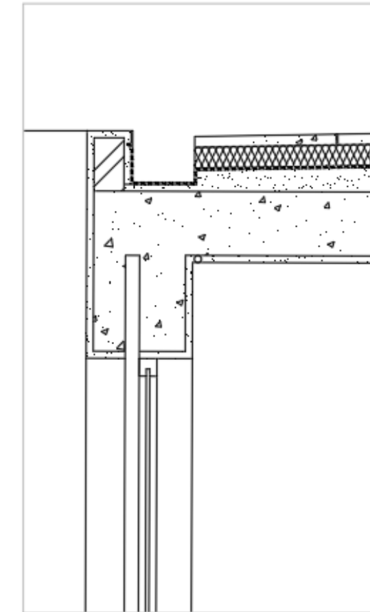
Pormenor cobertura - esc. 1:5
