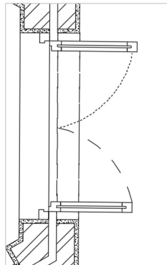
Pormenor - esc. 1:10
